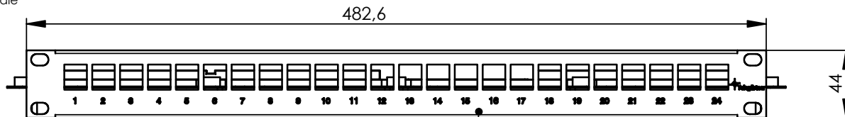
19" Modulträger inkl. Erdungs-Set / 19" frontplate incl. grounding kit
