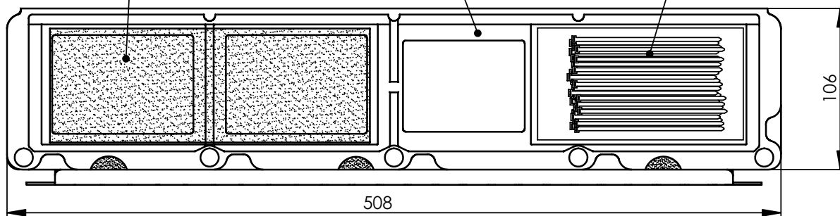
19" Modulträger inkl. Erdungs-Set / 19" frontplate incl. grounding kit
