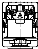
Montageausschnitt assembly cutout
