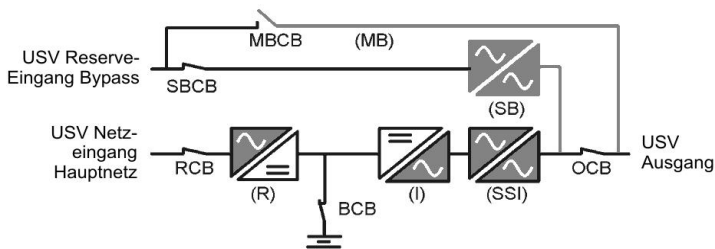
Abb. 3-2 Betriebsart: Normalbetrieb.
