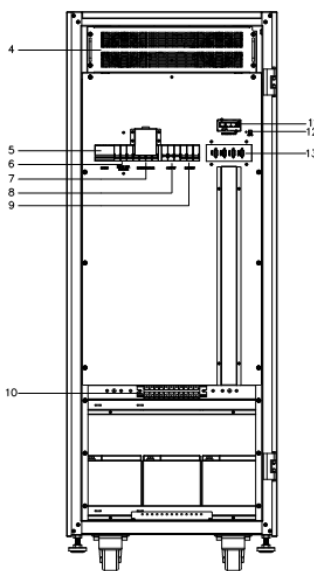
Abb. 3-8 USV-Frontansicht bei geöffneter Türe (10 – 20 kVA).
