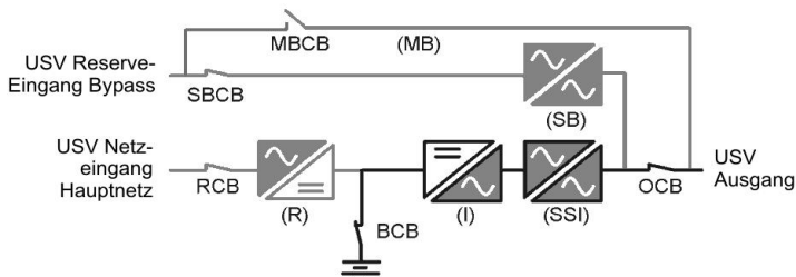
Abb. 3-3 Betriebsart: Autonomiebetrieb.
