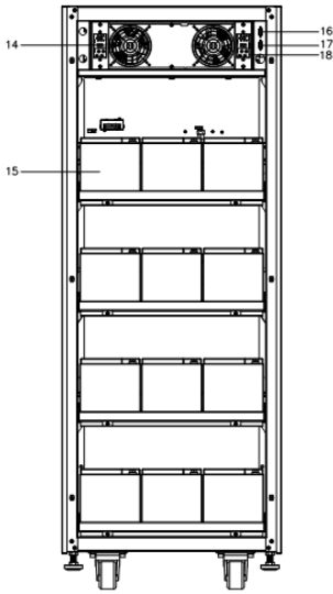
Abb. 3-9 USV-Rückansicht bei geöffneter Rückwand (10 – 20 kVA).
