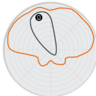
Abbildung 4. R750 2,4 GHz-Elevation-Antennenmuster
